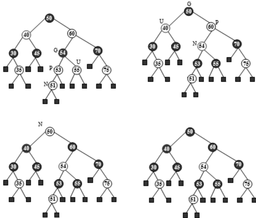
Insert 51
