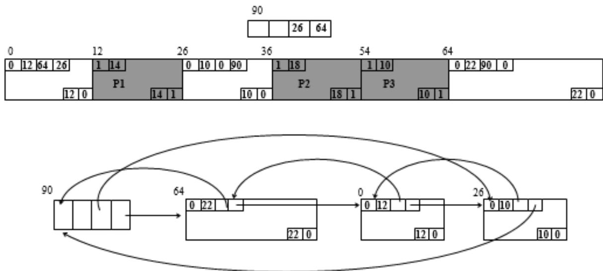
Figure 10.15 Free P4
