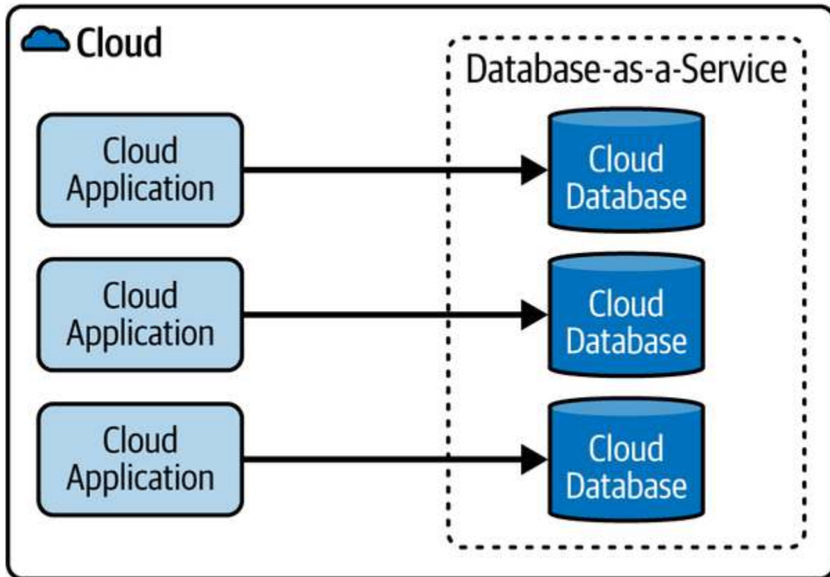
Figure 7-31. Database-as-a-Service
