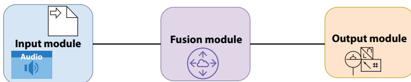
Figure 14.1 Multimodal AI.
