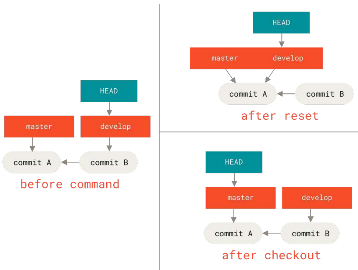
Figure 154. git checkout and git reset
